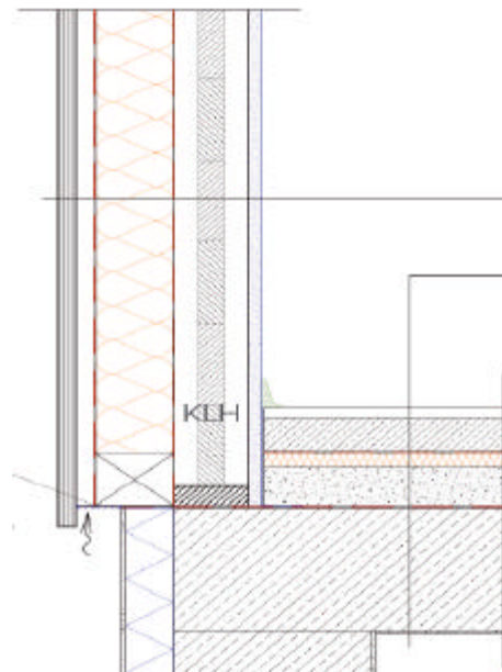
Dachaufsatz Aufbau
