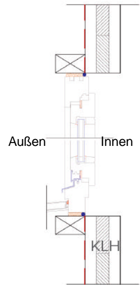
Fensterschnitt
